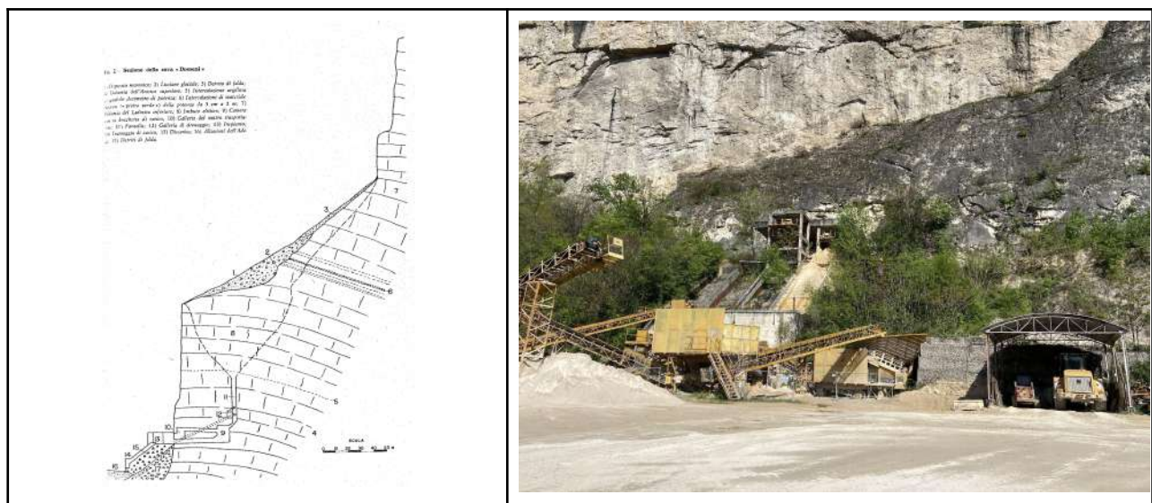
Fig. 4. A sinistra, una sezione geologica del versante su cui è impostata la miniera “Dossen”, con riportata la sagoma dell’imbuto roccioso col fornello sul fondo e il raccordo con la galleria che si sviluppa pressoché orizzontale fino allo sbocco dalla parete rocciosa (1976). A destra, una vista, dal piazzale di lavorazione, della struttura in cemento armato presente allo sbocco della galleria (2023).
