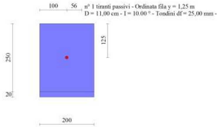
Fig. 2 - Prospetto del paramento con i tiranti
