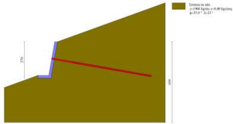
Fig. 7 - (Inviluppo)
