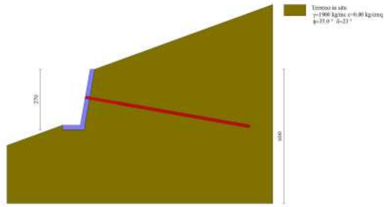
Fig. 3 - Stratigrafia
