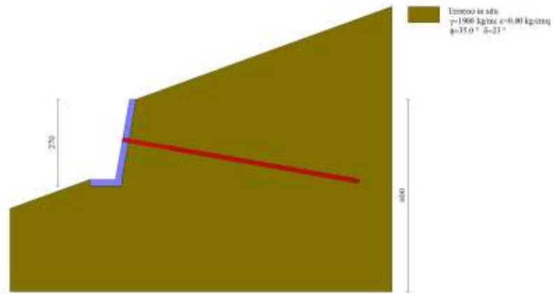
Fig. 9 - (Inviluppo)
