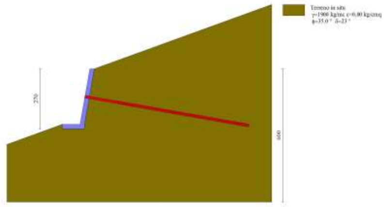
Fig. 8 - (Inviluppo)
