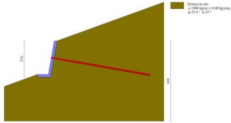
Fig. 6 - (Inviluppo)
