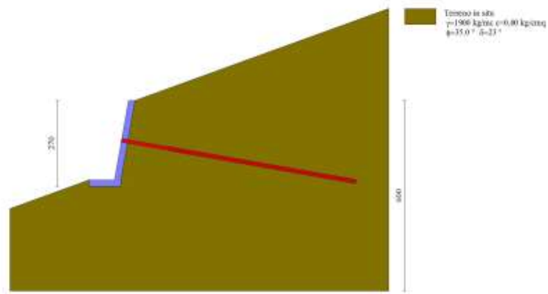
Fig. 5 - (Inviluppo)
