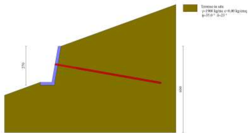
Fig. 11 - (Inviluppo)
