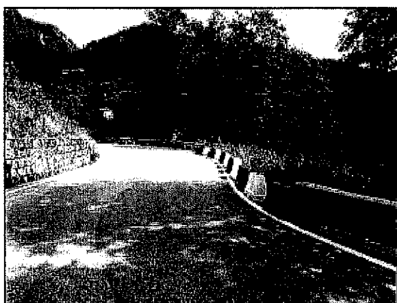
FOT.3 - Installazione barriere new Jersey fronte strada
