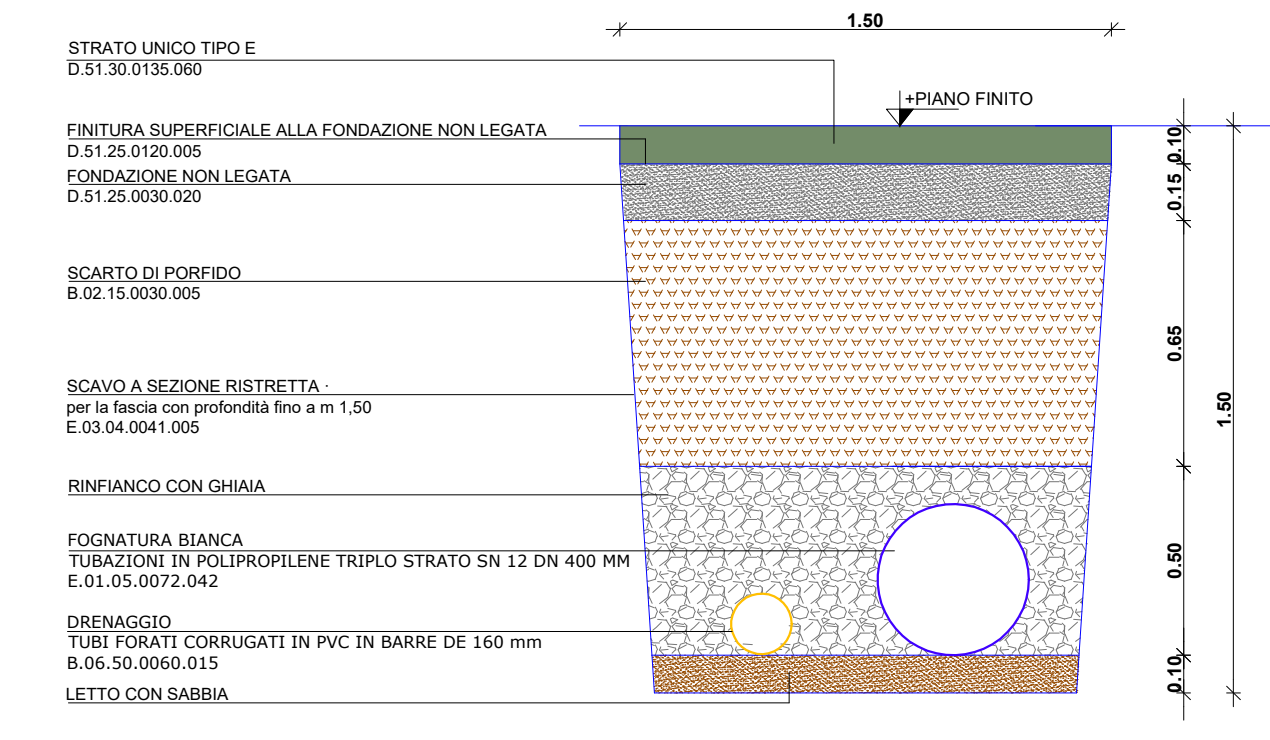
SEZIONE TIPO FOGNATURA BIANCA AL KM 0+600 CIRCA
