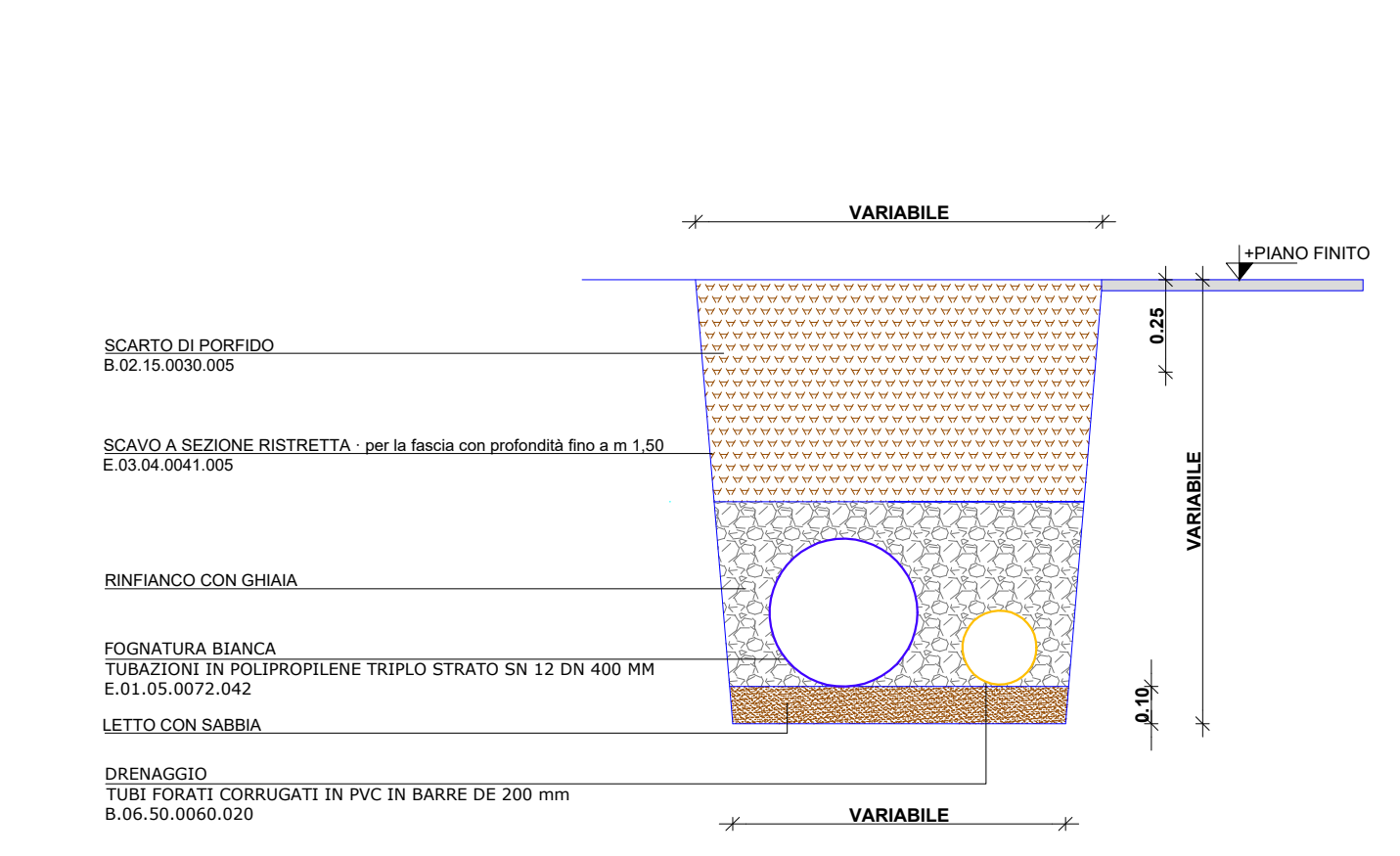
SEZIONE TIPO FOGNATURA BIANCA CON DRENAGGIO TRA IN KM 0+317 E IL KM 0+340 CIRCA
