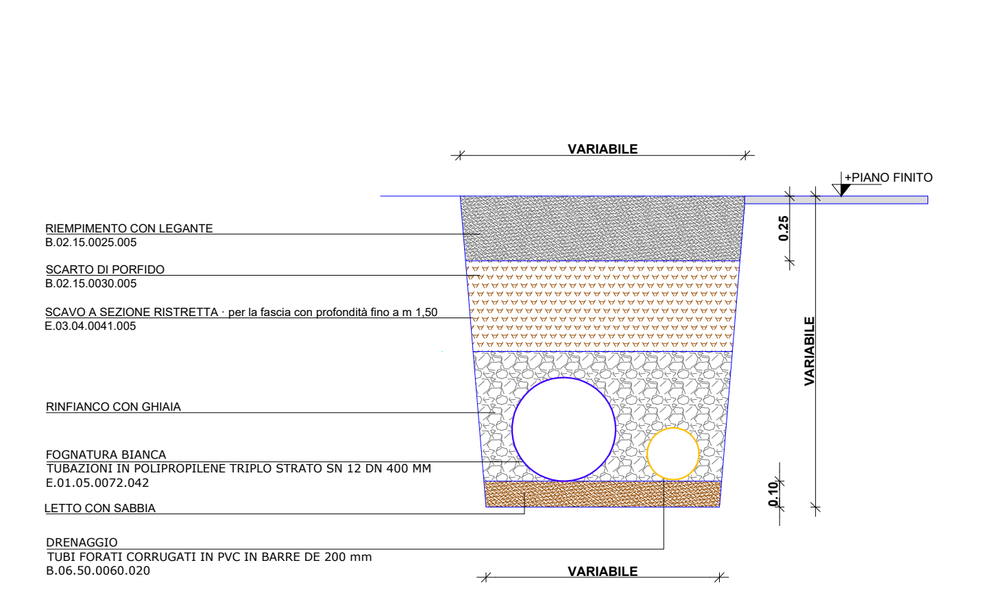
SEZIONE TIPO FOGNATURA BIANCA CON DRENAGGIO TRA IN KM 0+275 E IL KM 0+317 CIRCA
