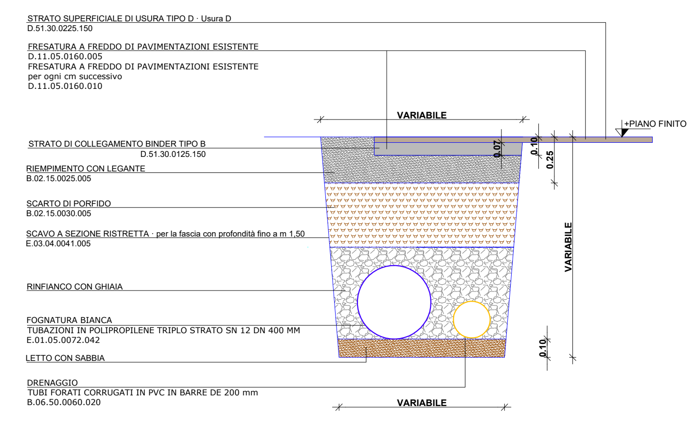
SEZIONE TIPO FOGNATURA BIANCA CON DRENAGGIO TRA IN KM 0+184 E IL KM 0+275 CIRCA
